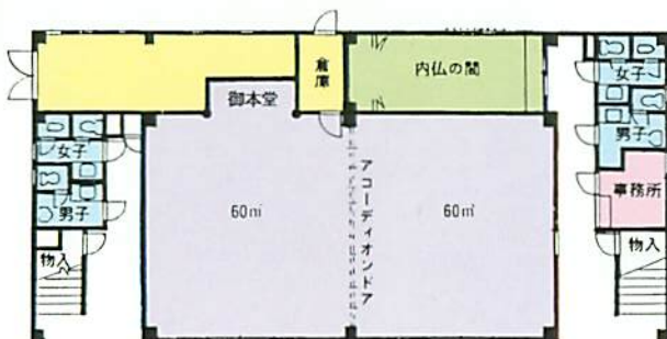
1階平面図
